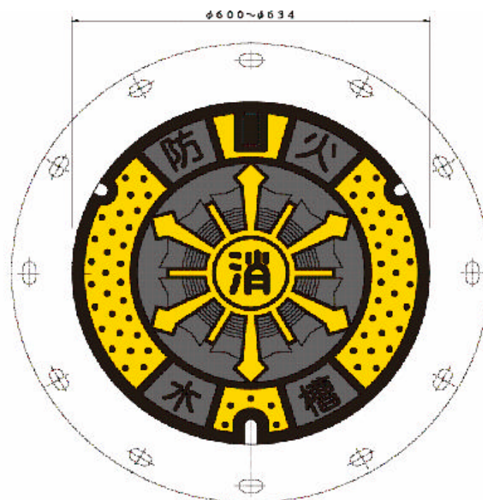
防火水槽鉄蓋図
